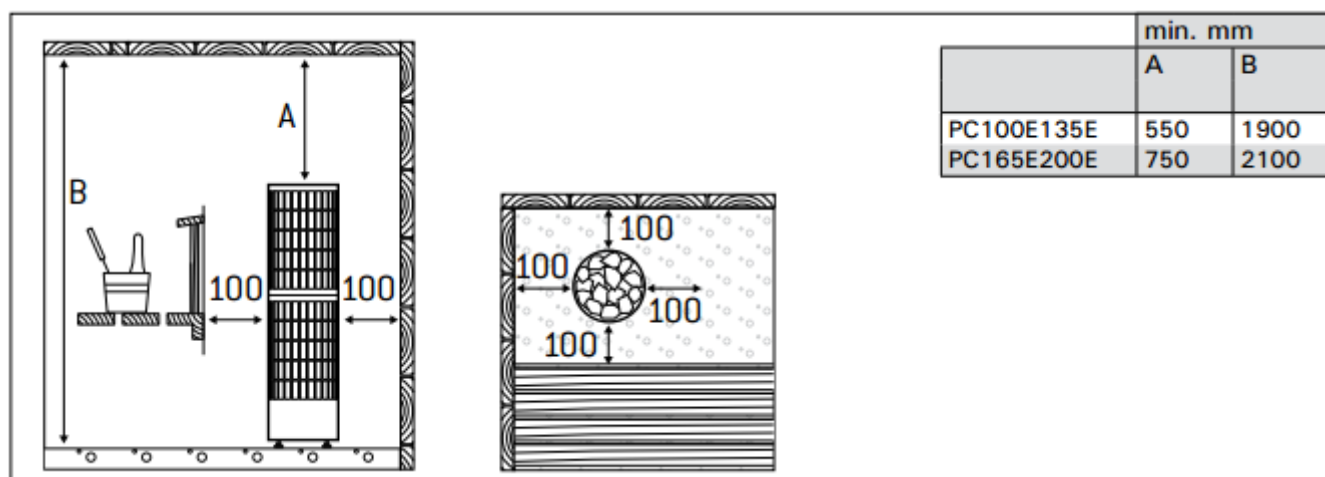
Rys. 6. Minimalne odległości instalacyjne (wymiar w milimetrach) Obrázek 6. Bezpečné vzdálenosti (všechny rozměry jsou uvedené v milimetrech)
